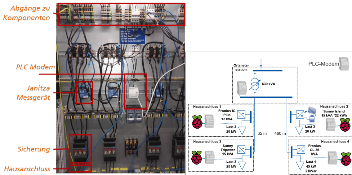
Abbildung 31: Aufbau BPL Vermessung
