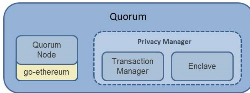
Abbildung 21: Darstellung der Komponenten eines Quorum Knotes
