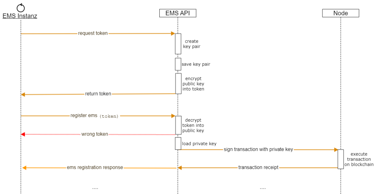
Abbildung 10: Anwendung mit Token-basierter Authentifizierung
