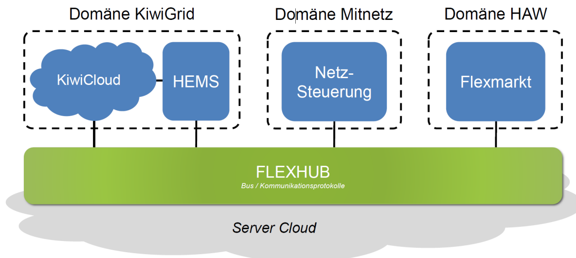
Abbildung 19: Erste monolithische Architektur zur Domänenabgrenzung.
