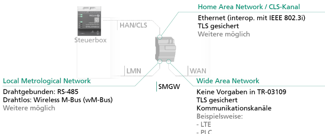
Abbildung 27: SMGW-Infrastruktur für den FlexHub
