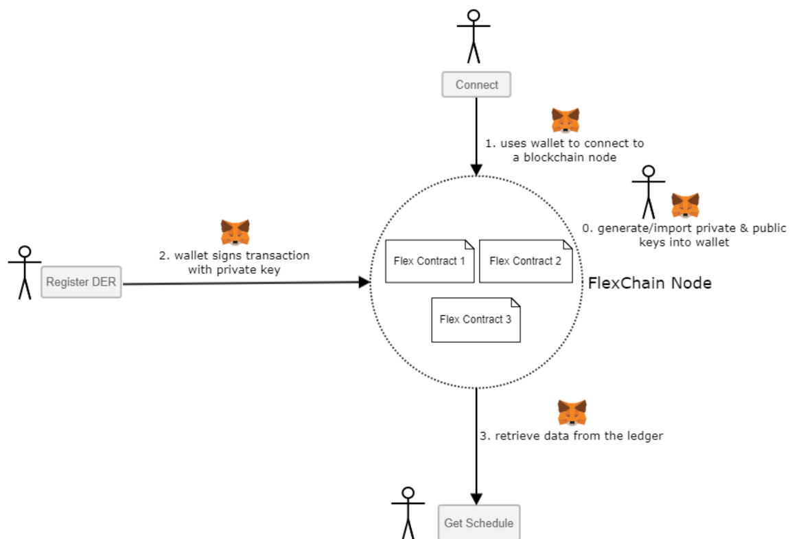
Abbildung 11: Ablauf des Authentifizierungsverfahrens mittels eines digitalen Wallet
