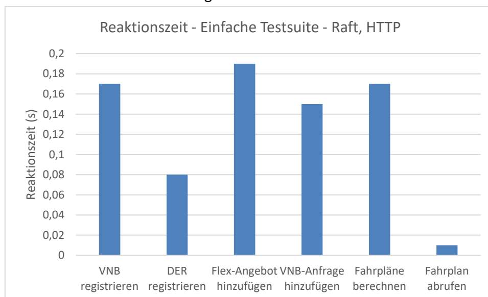
Abbildung 38: Reaktionszeiten der FlexChain Sandbox APIs (Raft) auf die Anfragen der "einfachen Testsuite"
