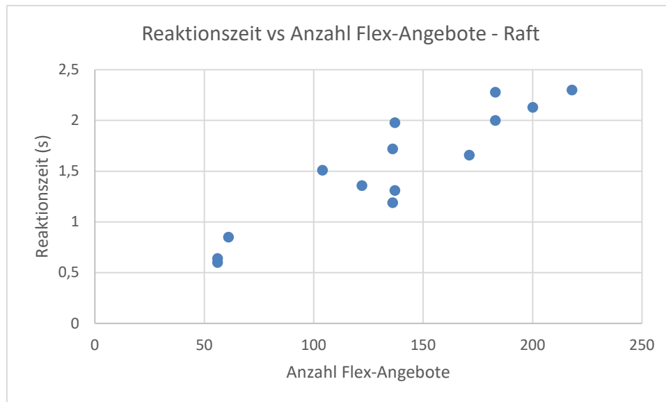
Abbildung 42: Die Reaktionszeit gegen die Anzahl der Flex-Angebot bei der FlexChain Sandbox APIs (Raft)
