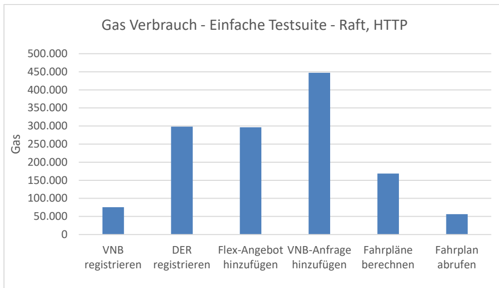
Abbildung 39: Gas Verbrauch der FlexChain Sandbox APIs (Raft) auf die Anfragen der "einfachen Testsuite"
