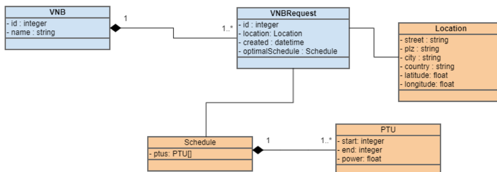
Abbildung 18: VNB- und VNBRequest Klassendiagramm
