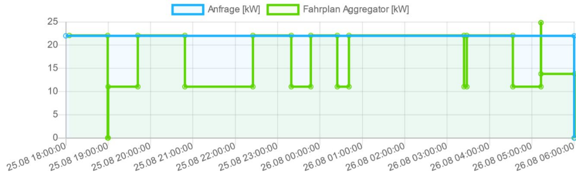
Abbildung 54: Screenshot NEMO.spot Weboberfläche Aggregationsanfrage und Lösung vom 25.08.2022
