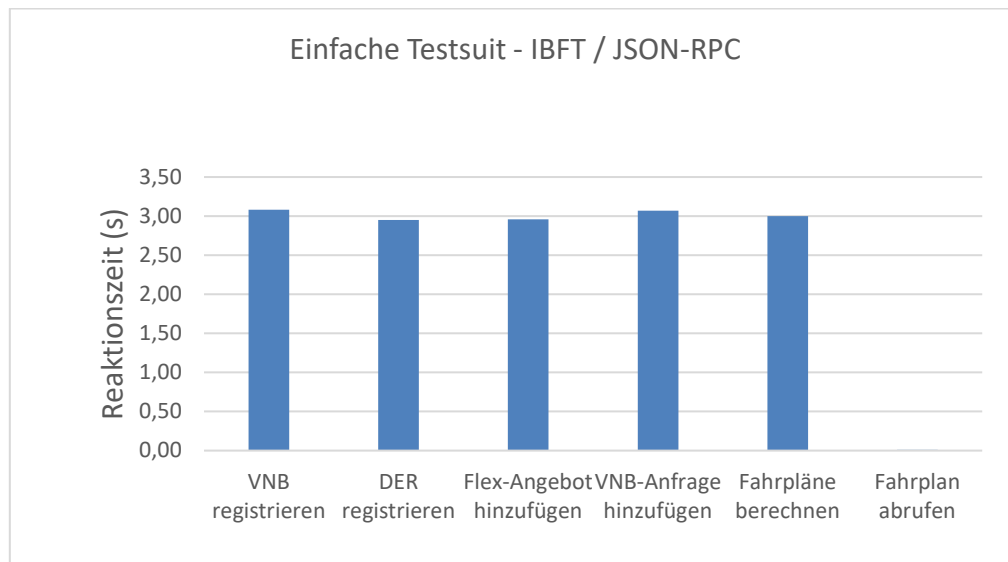
Abbildung 36: Die Reaktionszeiten der FlexChain Sandbox APIs (IBFT) auf die Anfragen der "einfachen Testsuite"
