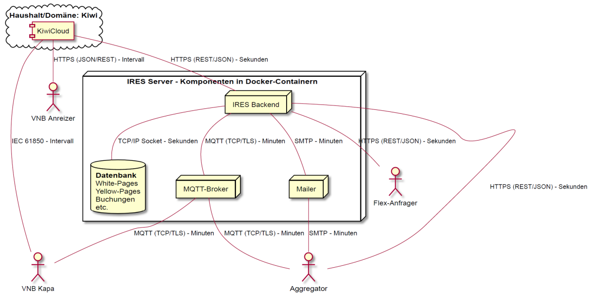
Abbildung 20: Architektur des Flexibilitätsregisters in einem verteilten Flexhub
