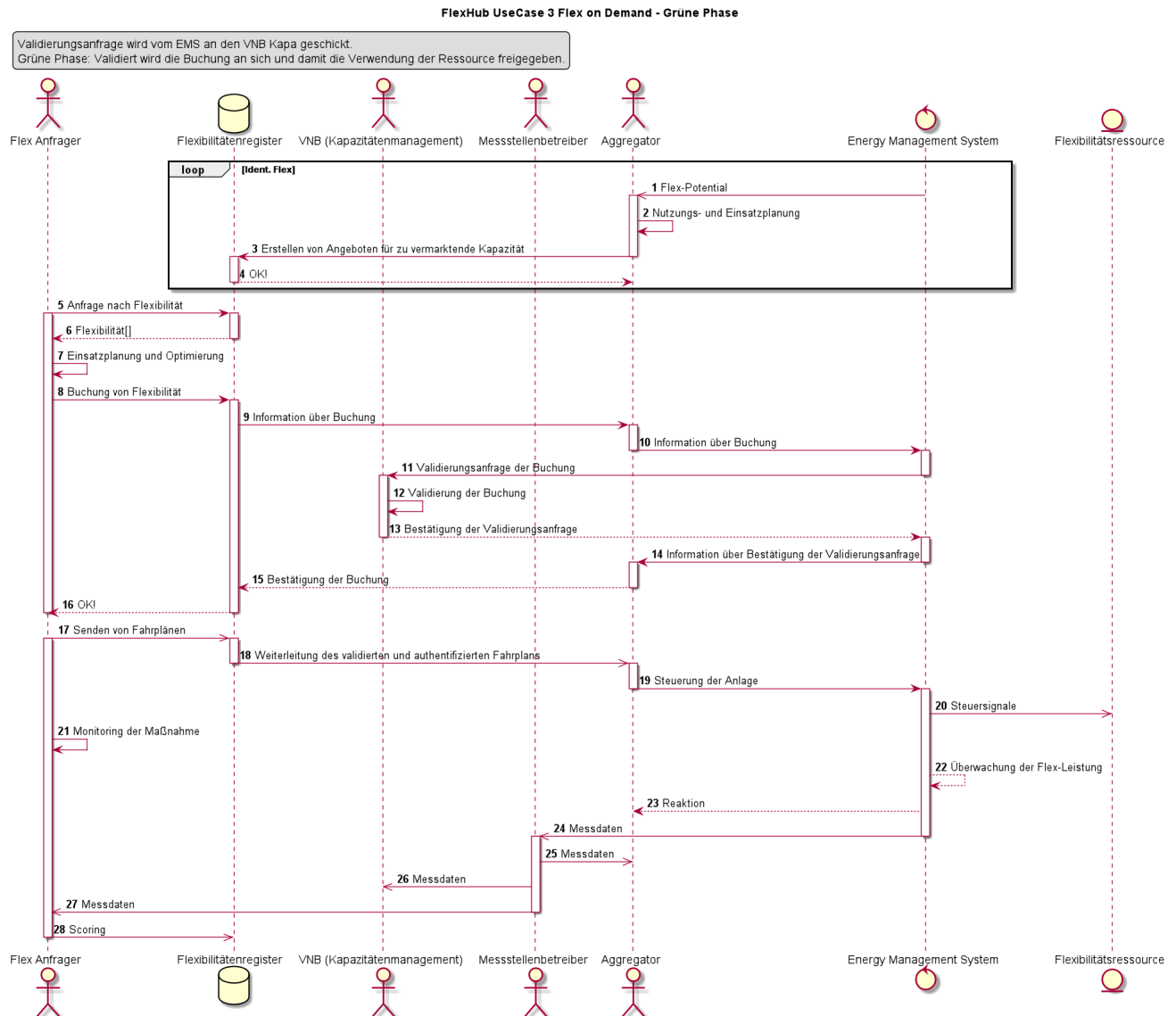
Abbildung 6: Flex on Demand Sequenzdiagramm – Vorwärtsweg, die Buchung wird Fahrplan-unabhängig bestätigt
