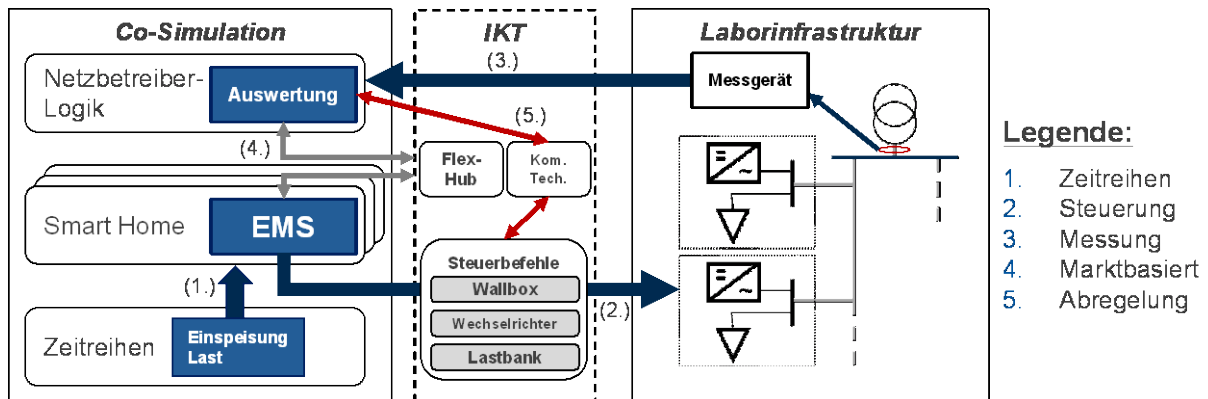
Abbildung II-47: Schematischer Aufbau der gesamten Laborinfrastruktur (Hard- und Software) [1]
