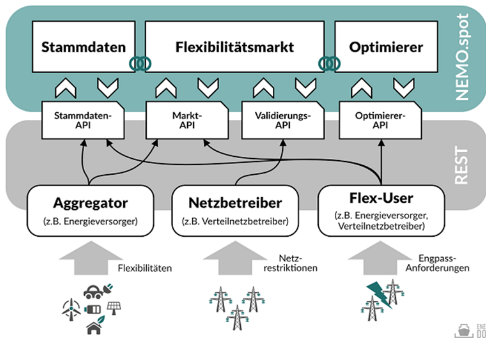
Abbildung 35: Architektur der NEMO.spot Plattform
