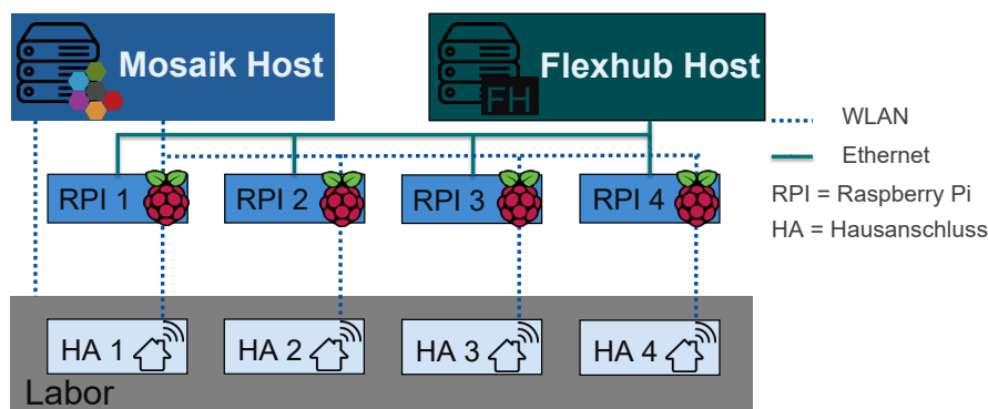
Abbildung II-48: Schematischer Aufbau der Kommunikationsschnittstellen
