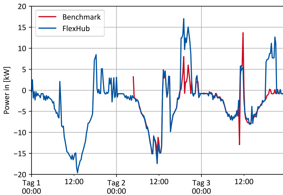
Abbildung II-53: Leistungsverlauf der ONS mit vier unterlagerten Hausanschlüssen
