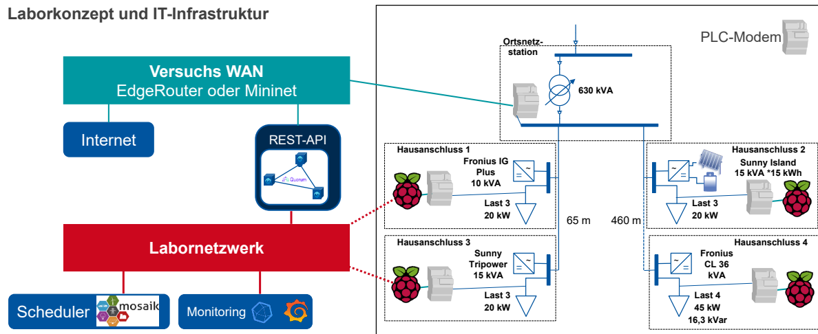
Abbildung II-51: Versuchsaufbau zur Untersuchung des blockchain-basierten FlexHub
