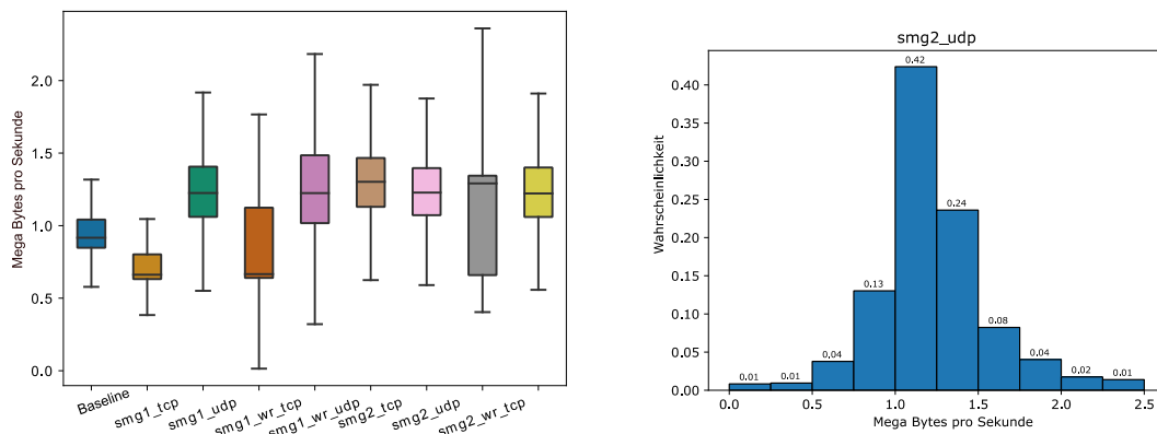
Abbildung 32: Vermessungsergebnisse BPL
