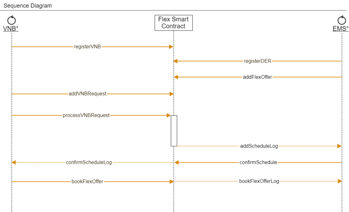
Abbildung 22: Sequenzdiagramm Interaktion mit dem Smart Contract gemäß Anwendungsfall 1
