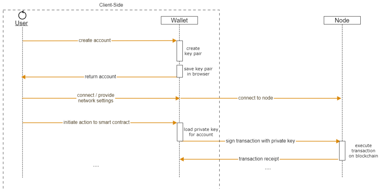
Abbildung 12: dApp mit Wallet Authentifizierung
