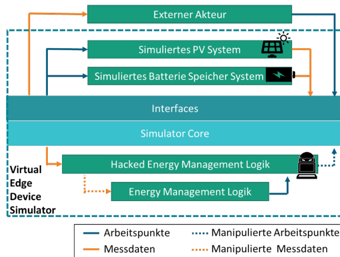
Abbildung 34: Aufbau Virtual Edge Device
