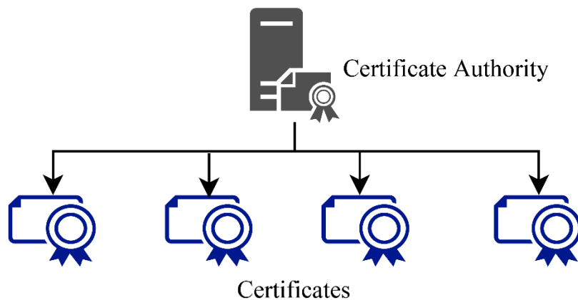
Abbildung 14: Hierarchische Vertrauensstruktur
