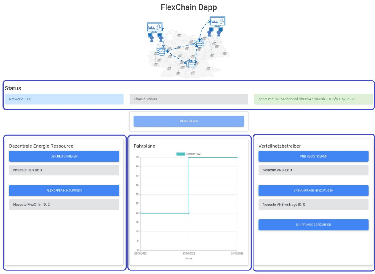
Abbildung 23: DApp Benutzeroberfläche mit Eingabe-Funktionen zur Flexibilitätsmarkt
