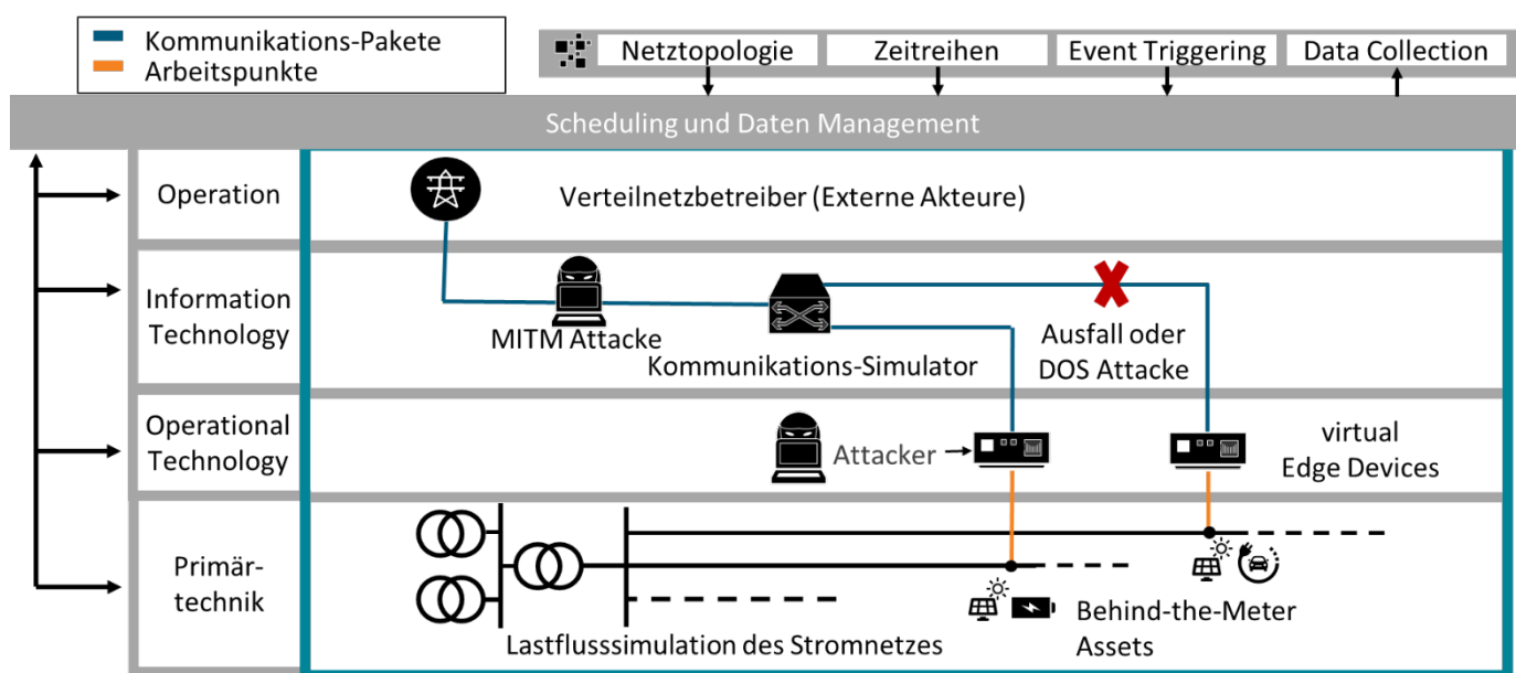
Abbildung 33: Aufbau Co-Simulation
