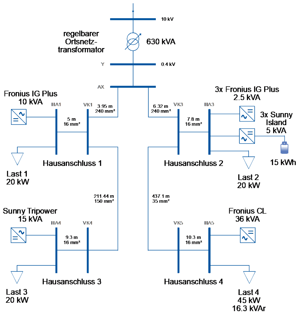
Abbildung II-49: Exemplarische Netztopologie [2]
