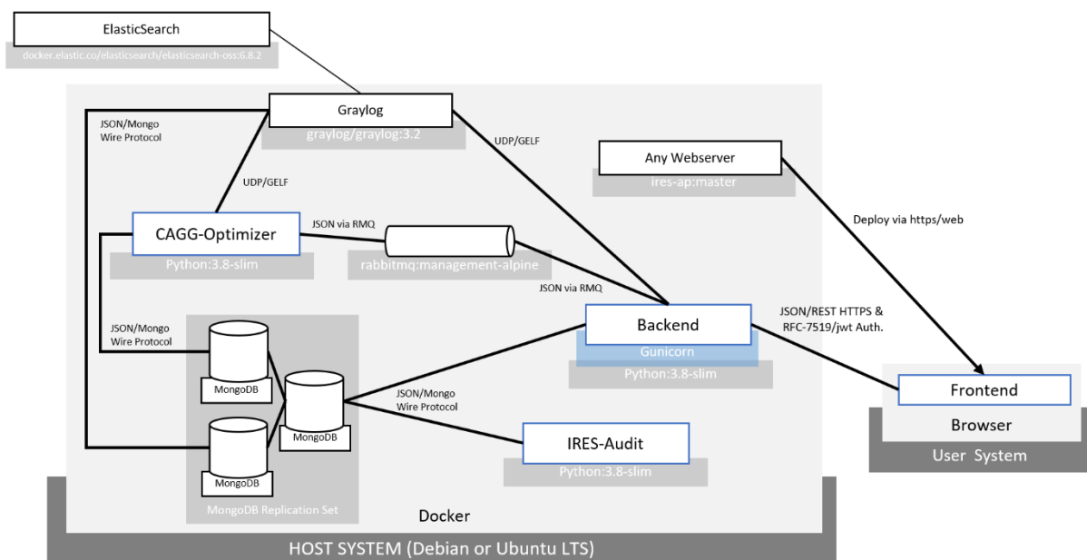
Abbildung 50: Deployment NEMO.spot Plattform Feldtest
