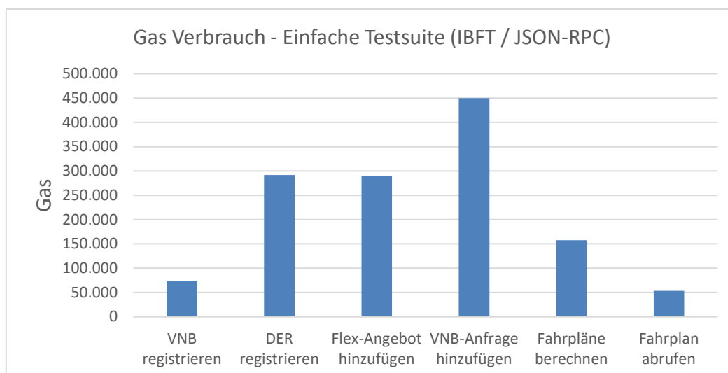
Abbildung 37: Gas Verbrauch der FlexChain Sandbox APIs (IBFT) auf die Anfragen der "einfachen Testsuite"
