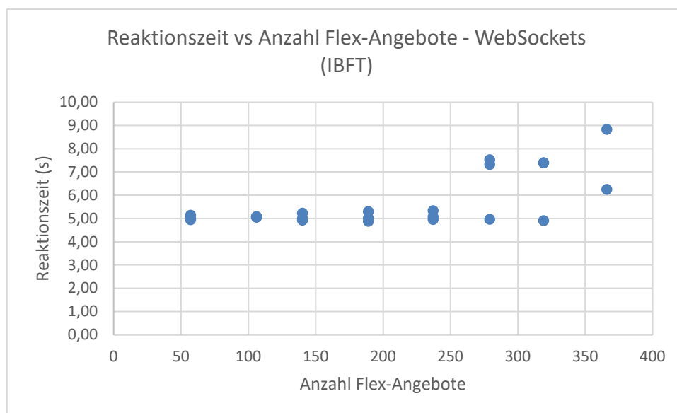
Abbildung 43: Die Reaktionszeit gegen die Anzahl der Flex-Angebot bei der WebSockets Verbindung (IBFT)
