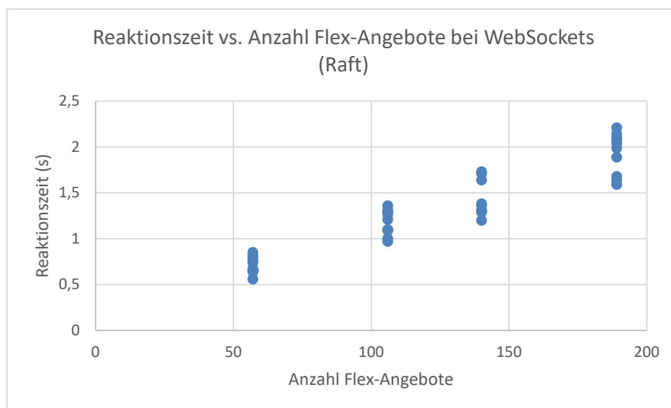
Abbildung 44: Die Reaktionszeit gegen die Anzahl der Flex-Angebot bei der WebSockets Verbindung (Raft)
