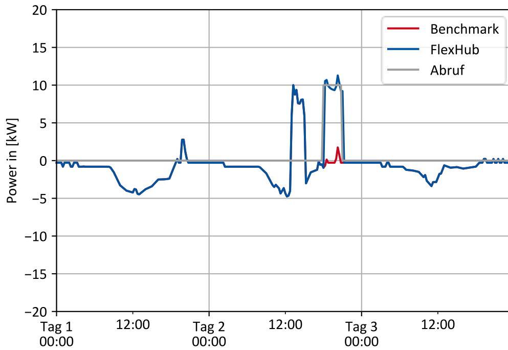
Abbildung II-52: Leistungsverlauf eines exemplarischen Hausanschlusses
